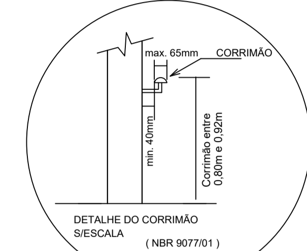
DETALHE 1
